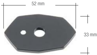
Plates for direction indicators Placas cubre intermitente PFK2 € 14,50 for 4 pieces 4 unidades
