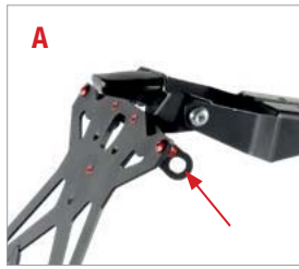
Hole for racing turn signals / Sujeción para intermitentes racing
